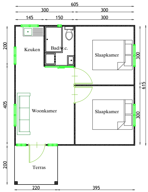
Plattegrond
