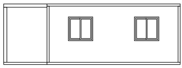
Rechterzijgevel
